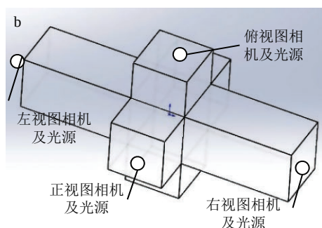
图 12 相机阵列
