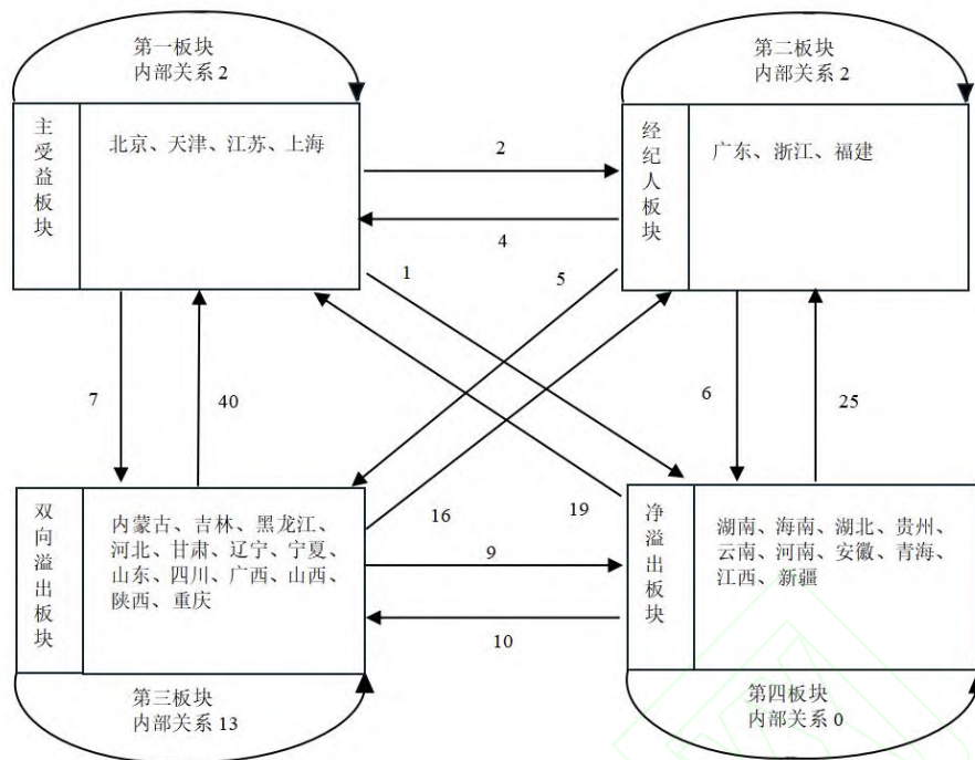
(b) 2022 年
