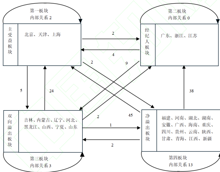
(a) 2010 年
